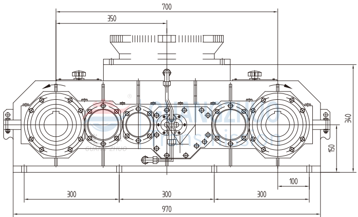
HL700-外形图
