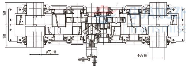
HL890-外形图
