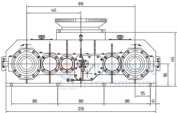
HL890-外形图
