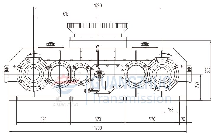
HL1230-外形图
