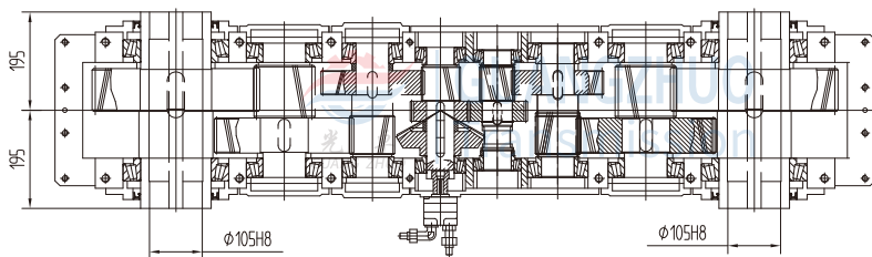
HL1230-外形图
