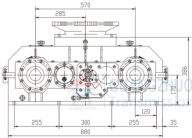
YHL570外形图
