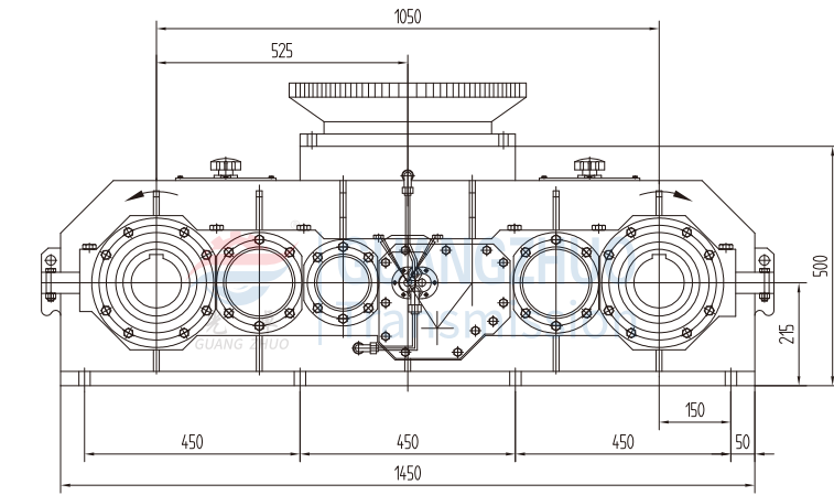
HL1050-外形图
