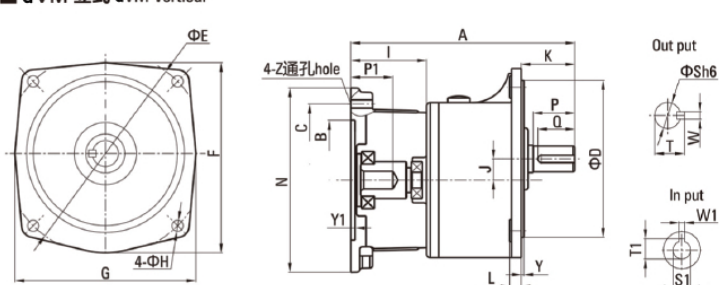
■ GVM 立式 GVM Vertical
