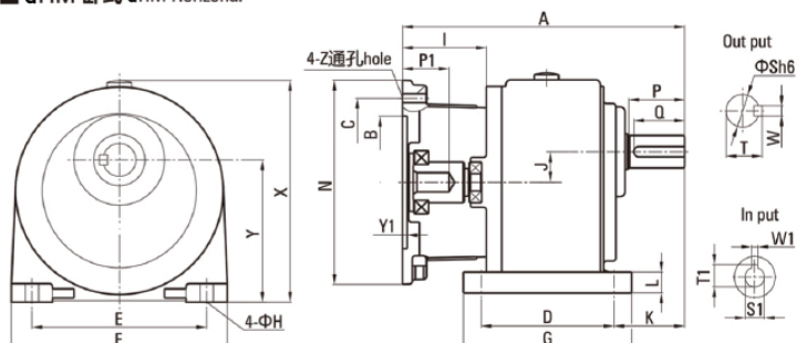
■ GHM 卧式 GHM Horizontal
